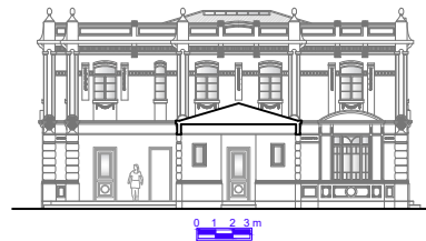
Elevação 02
