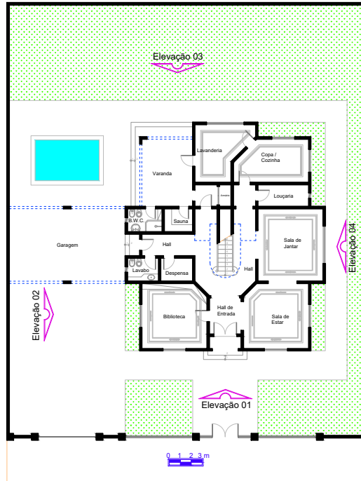
Térreo
