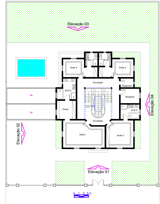
Superior
