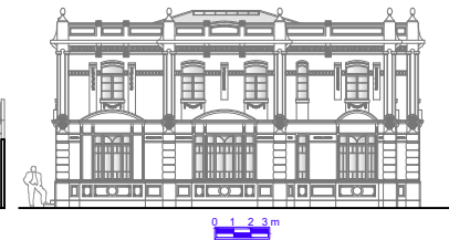
Elevação 04
