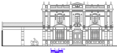
Elevação 01
